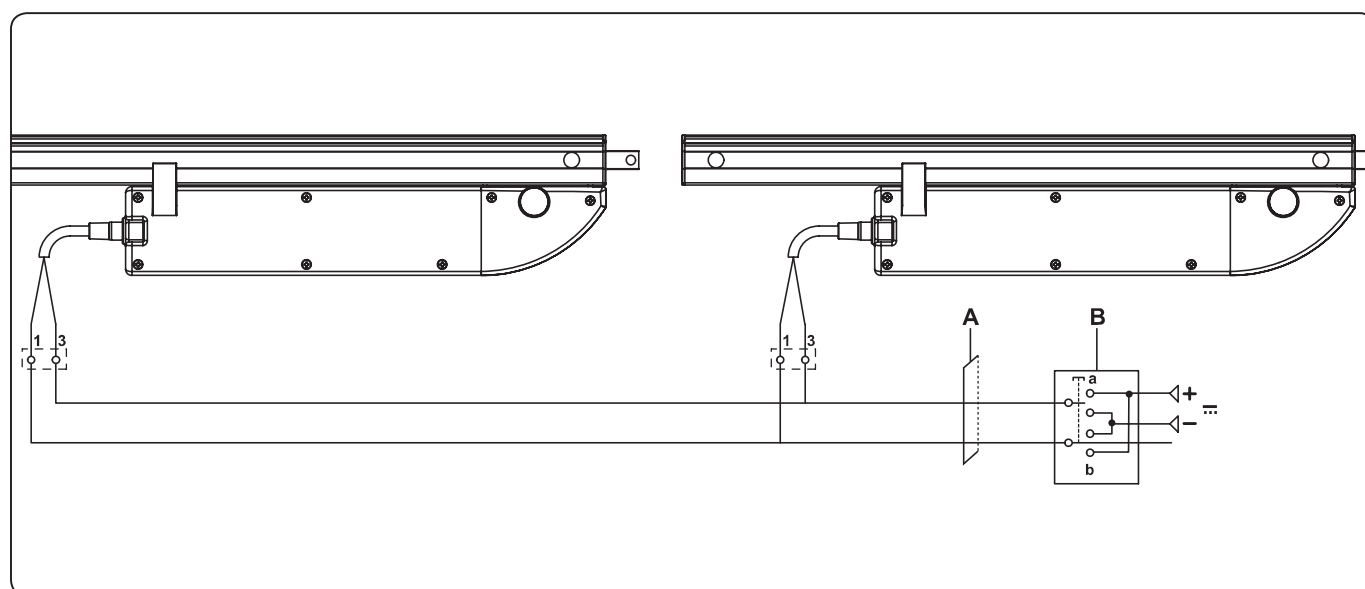
ⒸZ Zapojení více ovládacích mechanismů ⒸGB Connection of more than one actuator
