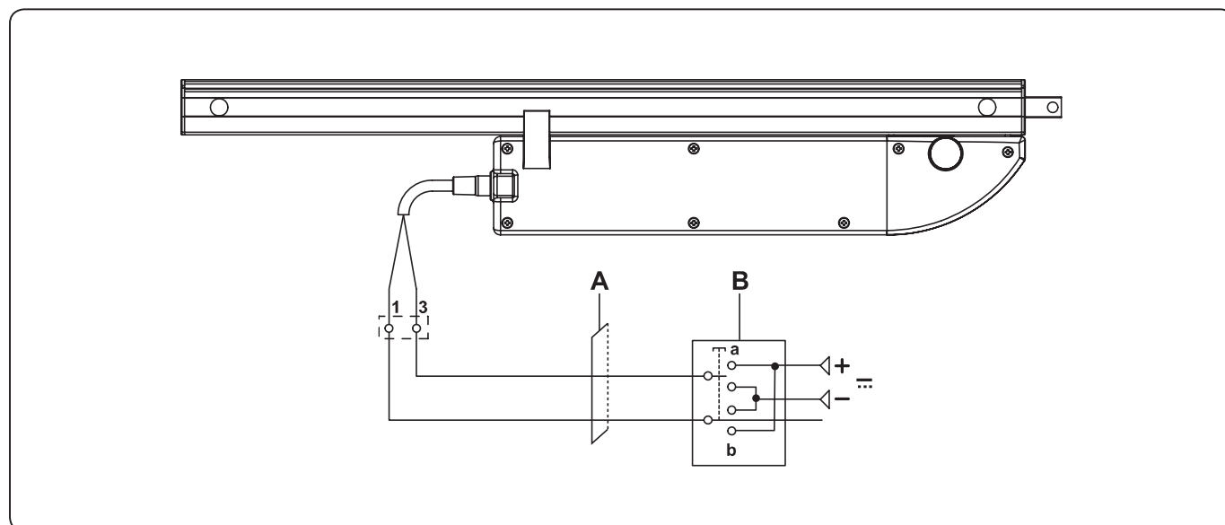
ⒸZ Zapojení jednoho ovládacího mechanismu ⒸGB Single connection
