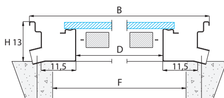
Příčný řez (X)
