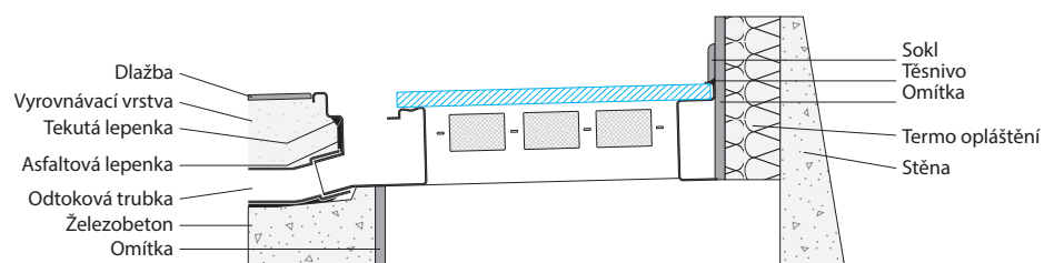
Schéma pokládky v blízkosti zdi
